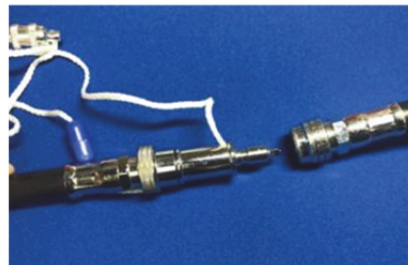
②次に、中圧アダプターに取り付けます
